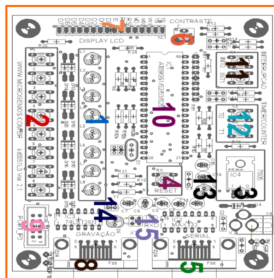
Figura 3.1 – Placa controladora do kit de desenvolvimento
