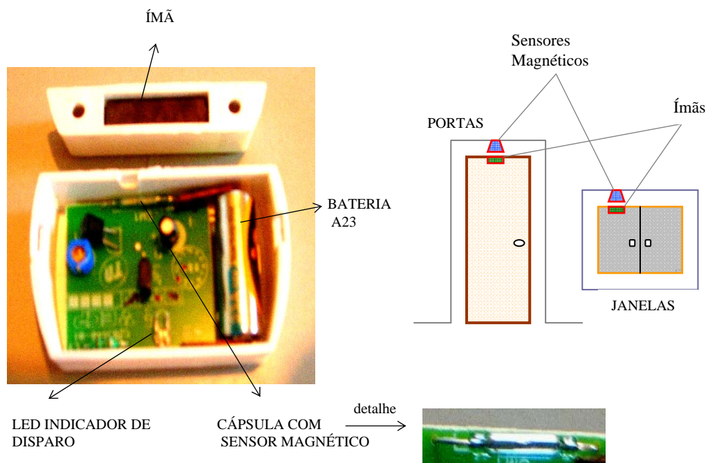
Figura 3.4 – Conjunto sensor magnético com ímã e o modo de instalação
