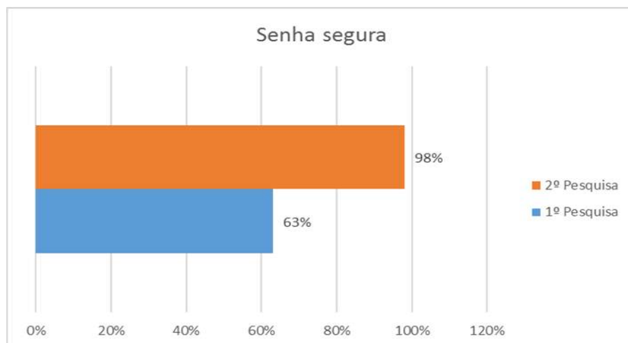
FIGURA 12 SENHA SEGURA
