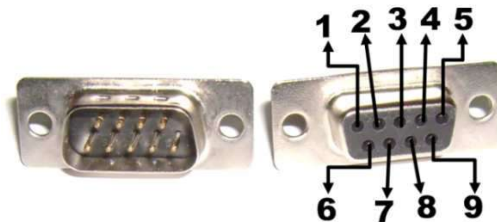
Figura 3.8 - Conector DB9 (FONTE: Braga, 2010, p. 53)
