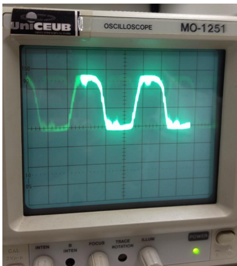
Figura 4.1 - Gráfico do sensor sendo acionado várias vezes.
