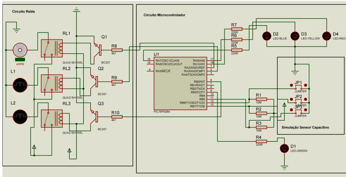
Figura 3.3 - Simulação dos circuitos no Proteus®.
