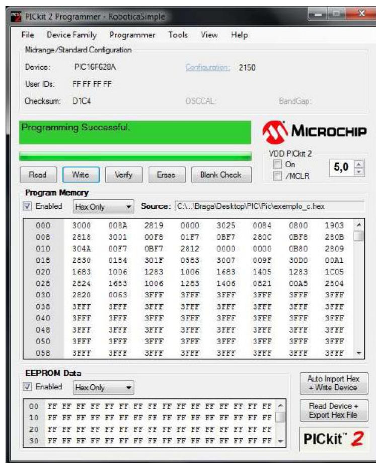
Figura 2.4 - PICKit2 Programmer.
