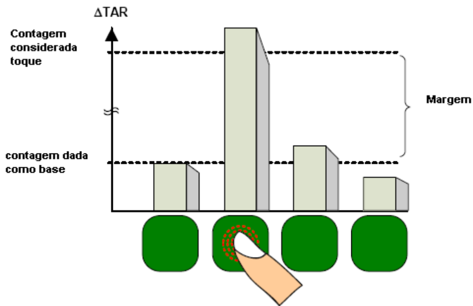
Figura 2.8 - Gráfico da capacitância do sensor capacitivo. (FONTE: Newton C. Braga, 2007)
