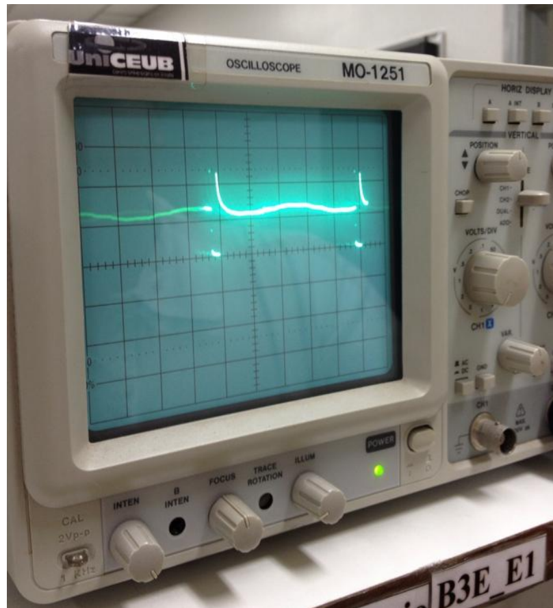
Figura 4.2 - Gráfico de carga e descarga do sensor.
