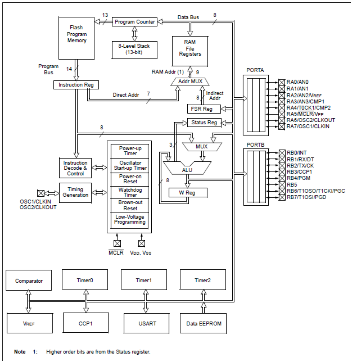
Figura 2.1 - Diagrama de Blocos do PIC16F628A.
