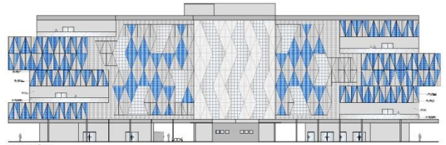
ELEVACÃO 2
