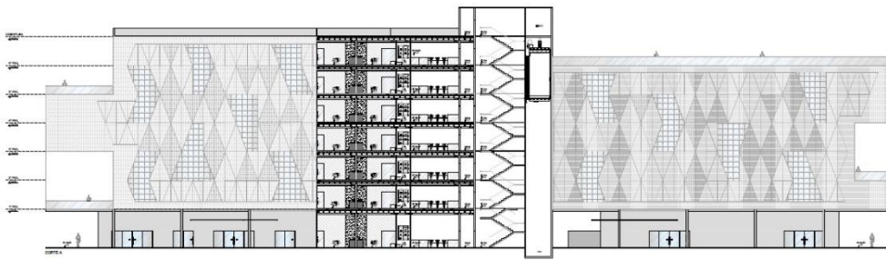
CORTE A
