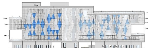
ELEVACÃO 3
