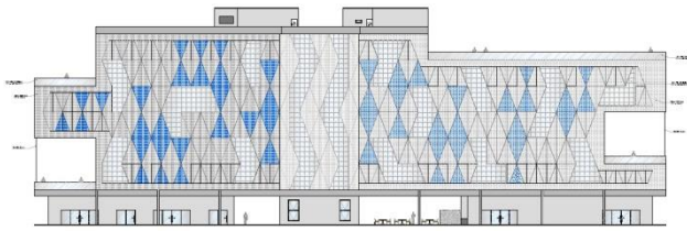
ELEVACÃO 1
