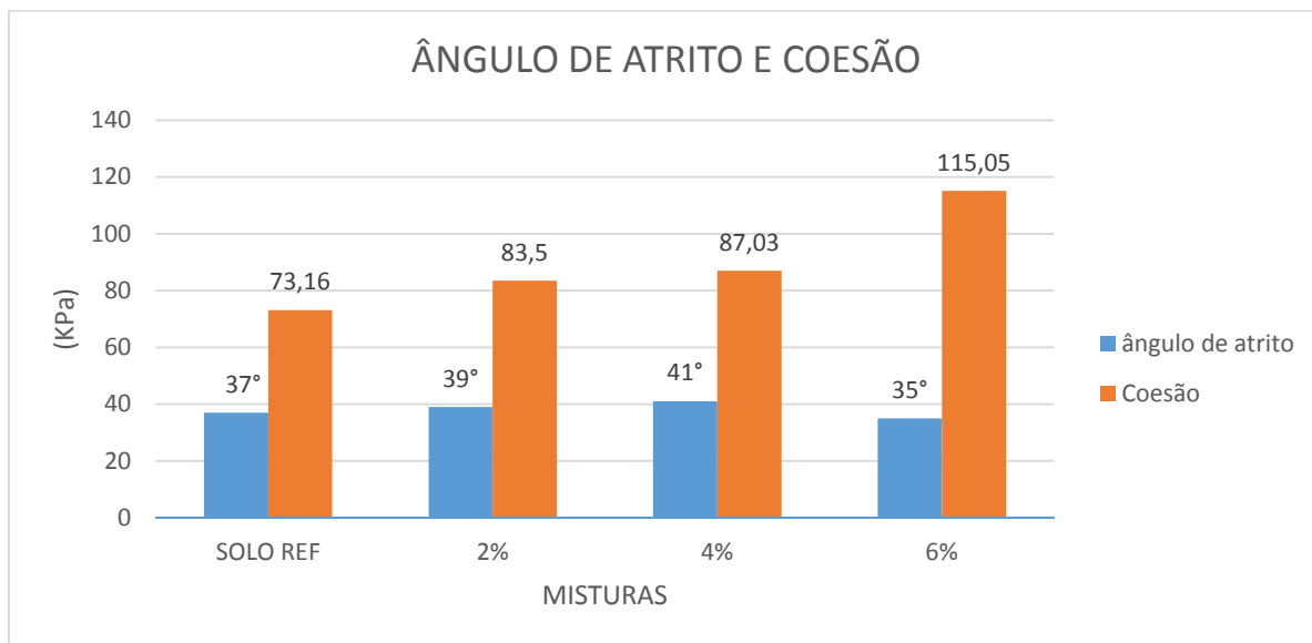
Gráfico : 17 – comparativo entre o ângulo de atrito e a coesão das amostras
