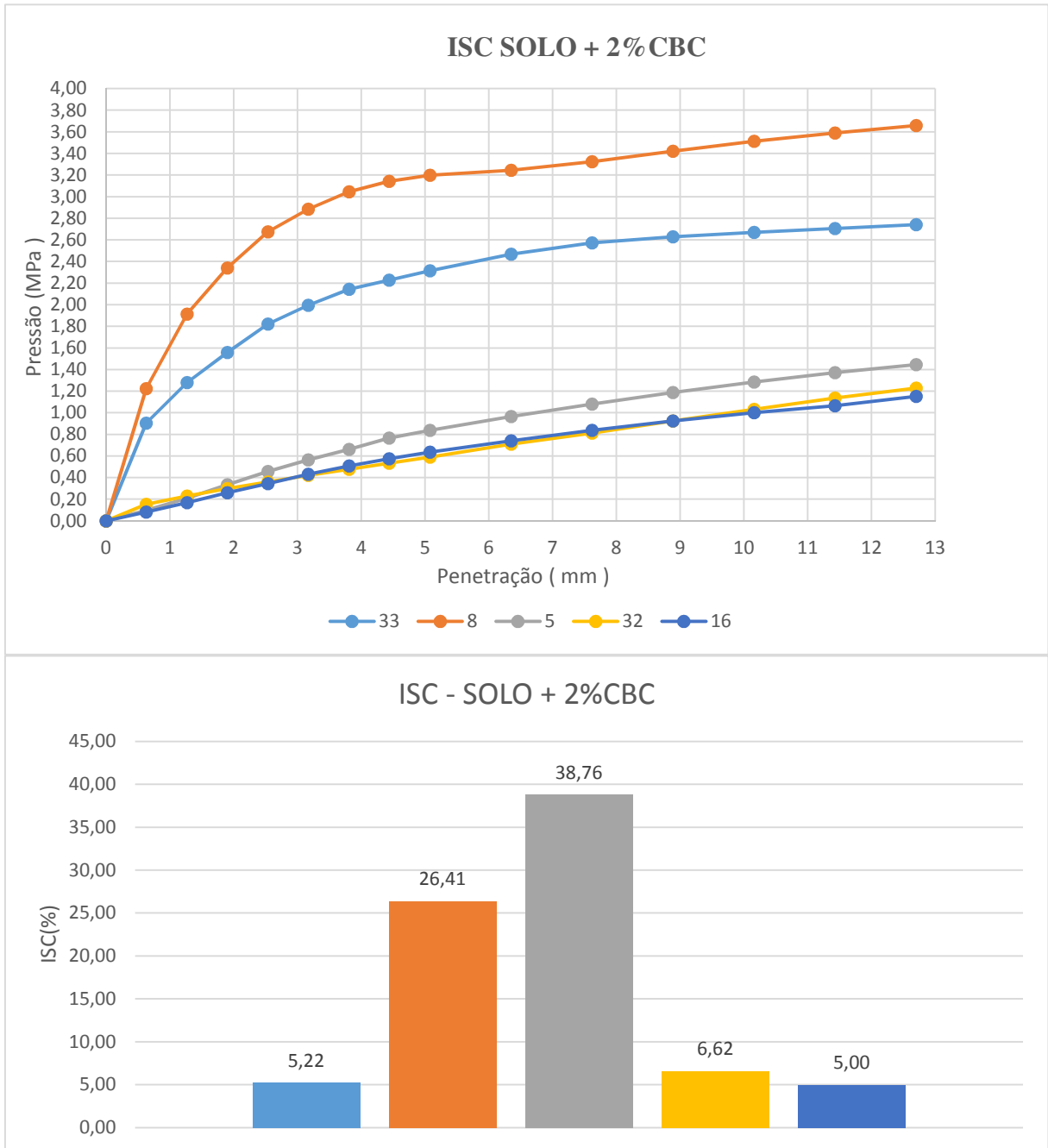
Gráfico : 9 - ISC solo +2% CBC
