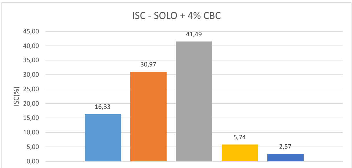
Gráfico : 10 - ISC solo +4% CBC
