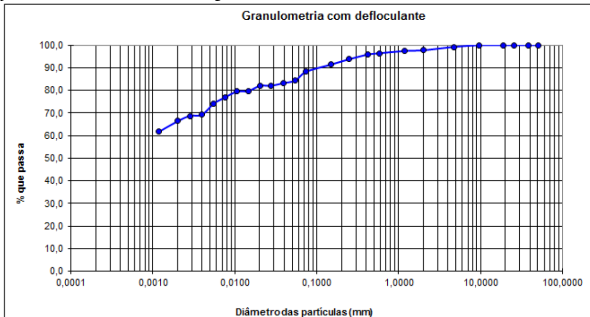
Gráfico : 1 – curva granulométrica
