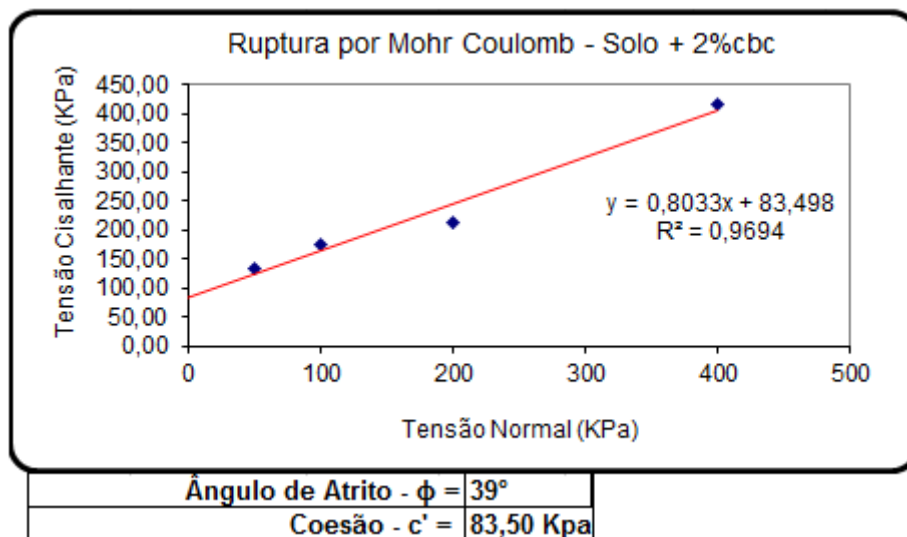
Gráfico : 14– cisalhamento solo + 2% CBC
