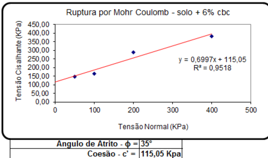
Gráfico : 16- cisalhamento solo + 6% CBC
