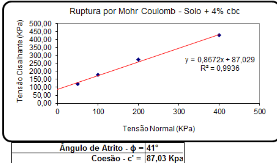
Gráfico : 15- cisalhamento solo + 4% CBC
