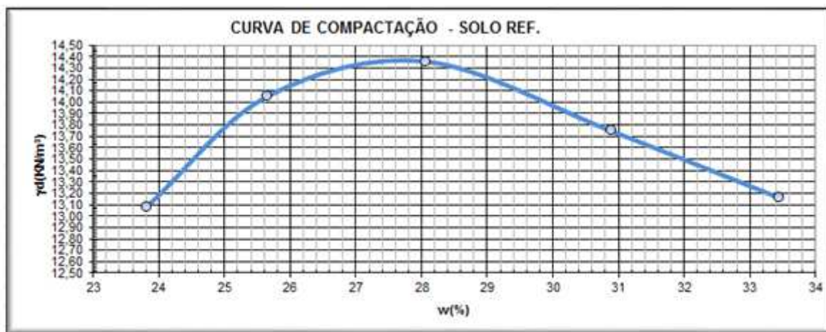
Gráfico : 2 – curva solo de referência
