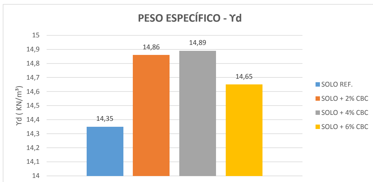
Gráfico : 7- comparativo entre os pesos específicos das amostras
