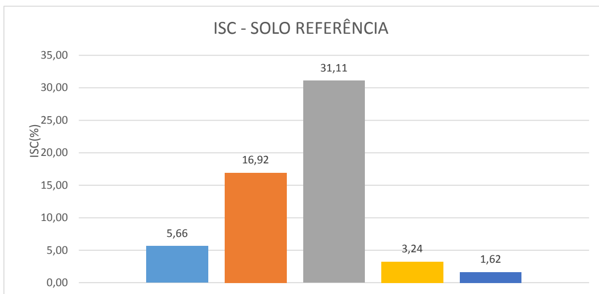
Gráfico : 8 – ISC solo de referência
