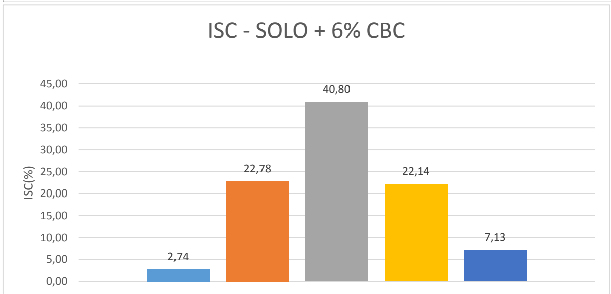
Gráfico : 11 - ISC solo +6% CBC
