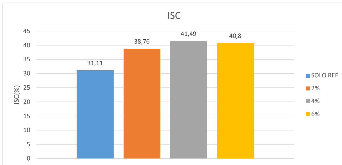
Gráfico : 12 – comparativo ISC das amostras
