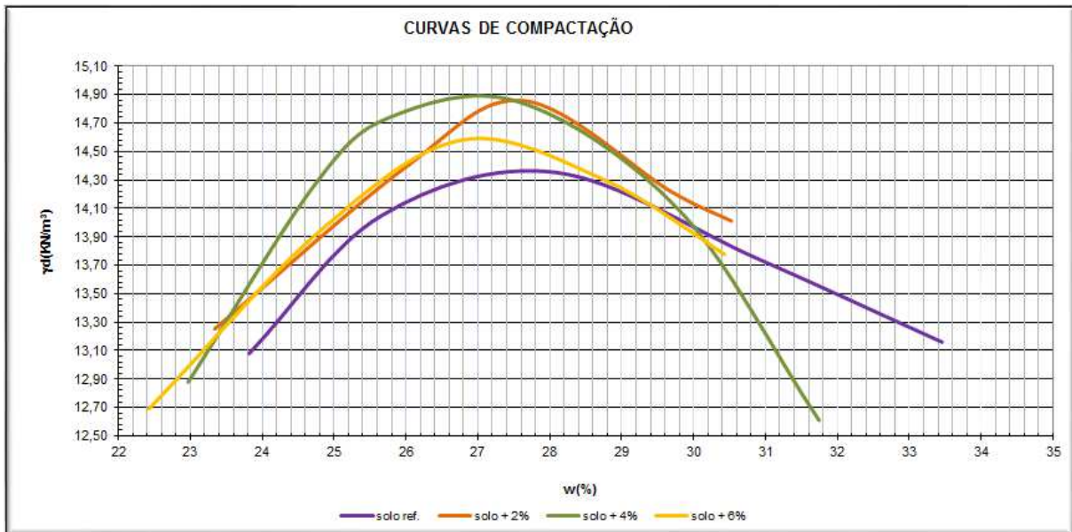
Gráfico : 6 – comparativo entre as curvas de compactação
