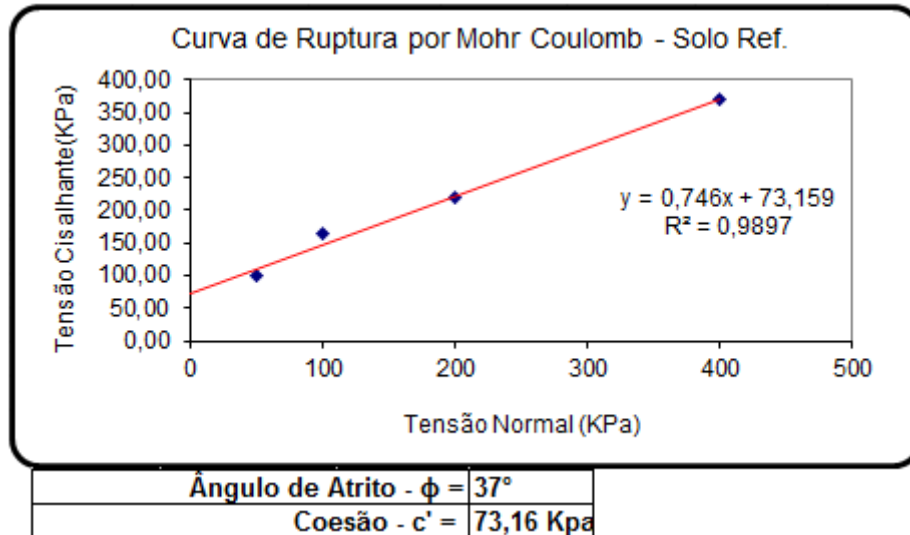
Gráfico : 13 – cisalhamento solo de referência
