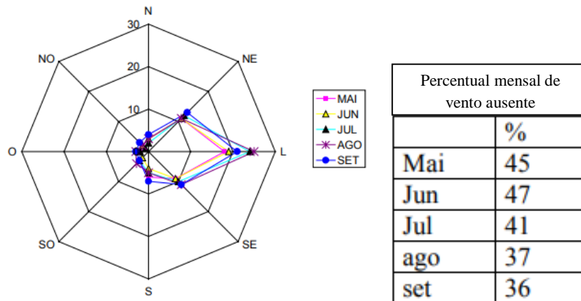
Figura 10 - Direção dos ventos no período seco - Brasília.
