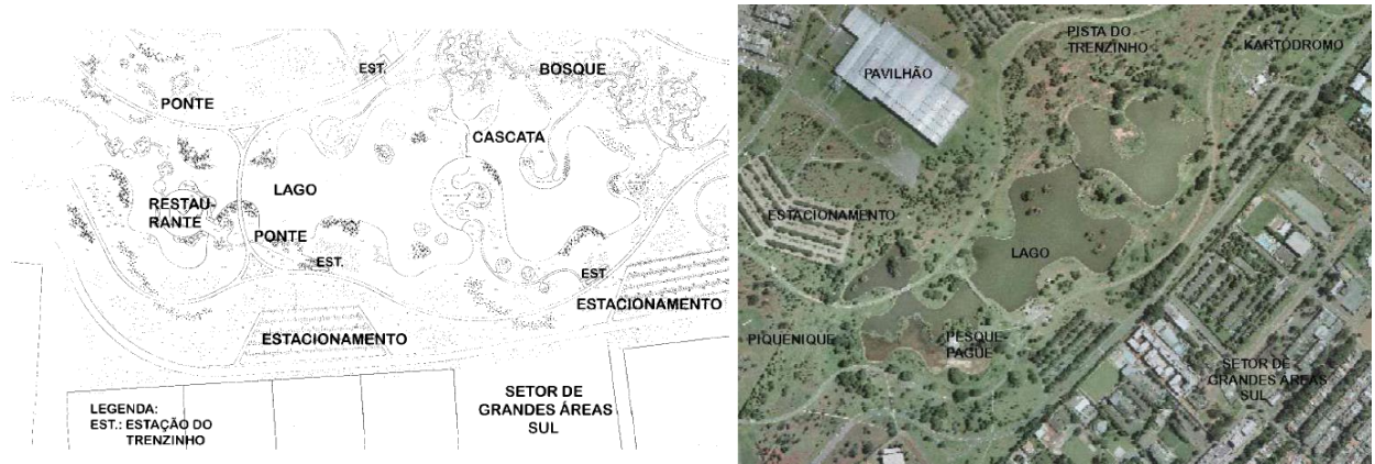
Figura 19 – Zona do Lago - projeto x construído.
