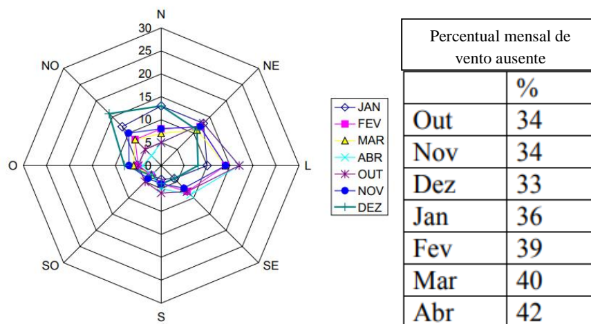
Figura 9 - Direção dos ventos no período quente e úmido - Brasília.
